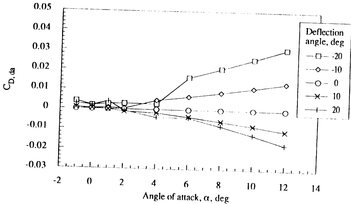
(d) Mach number = 1.5
