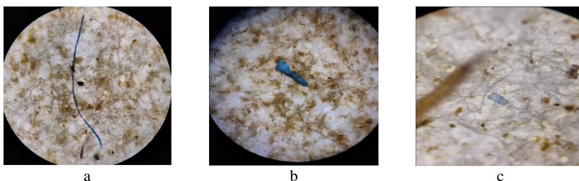
Gambar 2. Jenis mikroplastik yang ditemukan pada sampel air laut dengan tipe fiber (a), fragmen (b), film (c)
