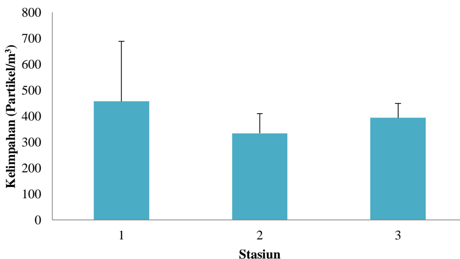
Gambar 1. Kelimpahan mikroplastik antar stasiun
