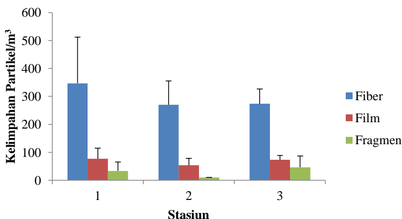
Gambar 3. Rata-rata kelimpahan mikroplastik antar stasiun berdasarkan jenis mikroplastik sampel air laut
