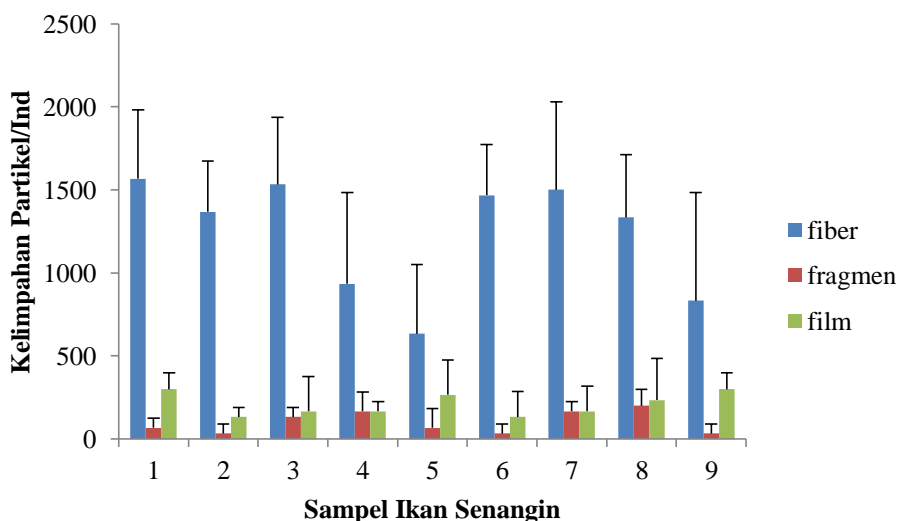
Gambar 4. Kelimpahan jenis mikroplastik sampel ikan senangin
