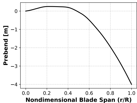
(d) Prebend
