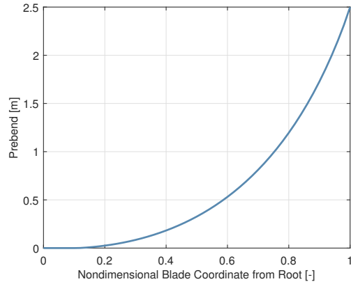
(f) Prebend
