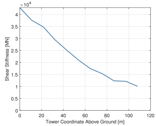
(d) Shear stiffness distribution
