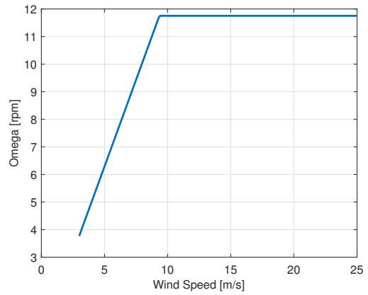
(d) Rotor speed
