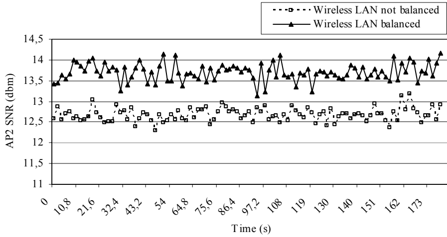
Figure 14 AP2 SNR
