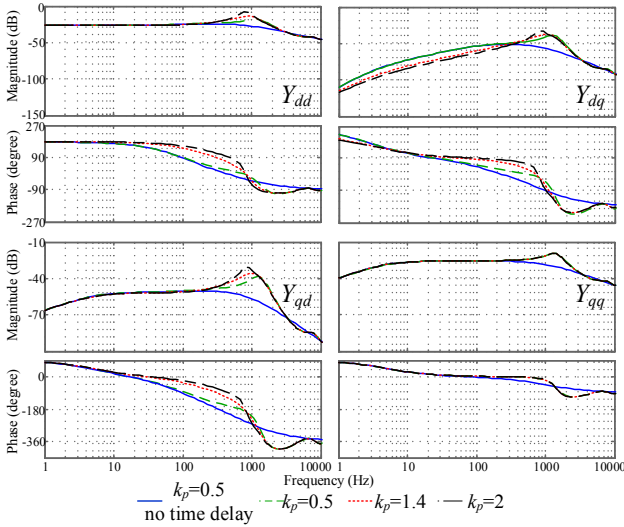
Fig. 9. Input admittance \mathbf{Y}_{cl} of rectifier mode represented in the dq -frame.
