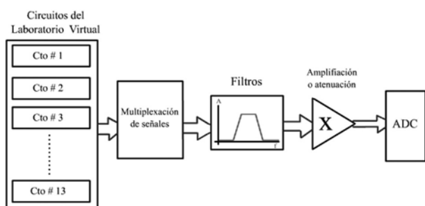
Figura 2. Diagrama de bloques de la selección y adecuación de señales.
