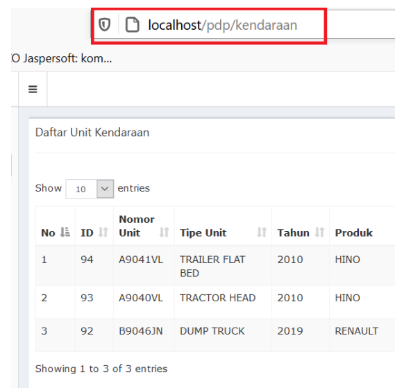
Fig. 11: Menu Kendaraan
