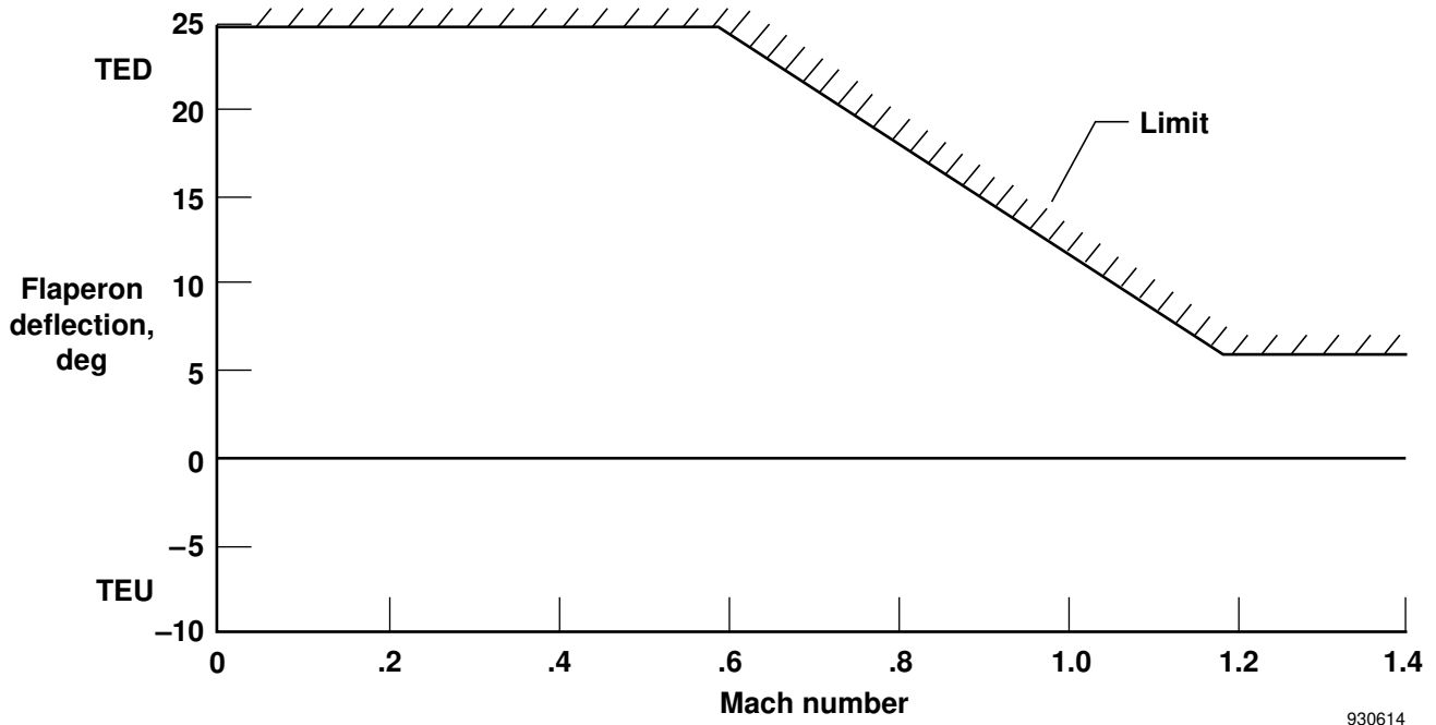
(b) Flaperon.
