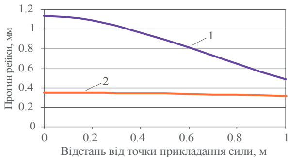
Рис. 6. Прогин рейки по довжині:
