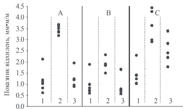
Рис. 3. Показник відхилення у вертикальній площині: 2 – в зоні переїзду; 1, 3 – на відстані 100 м до і після переїзду відповідно; A, B, C – ділянки з вантажонапруженістю 75, 72 і 84 млн ткм/км бруто
