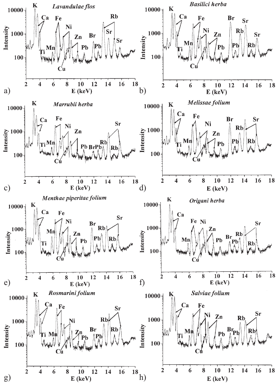
Fig. 1. EDXRF Spectra of ashed herbs samples obtained from plants of the family Lamiaceae : a) Lavandulae flos ; b) Basilici herba ; c) Merrubii herba ; d) Melissae folium ; e) Menthae piperitae folium ; f) Origani herba ; g) Rosmarini folium ; h) Salviae folium .
