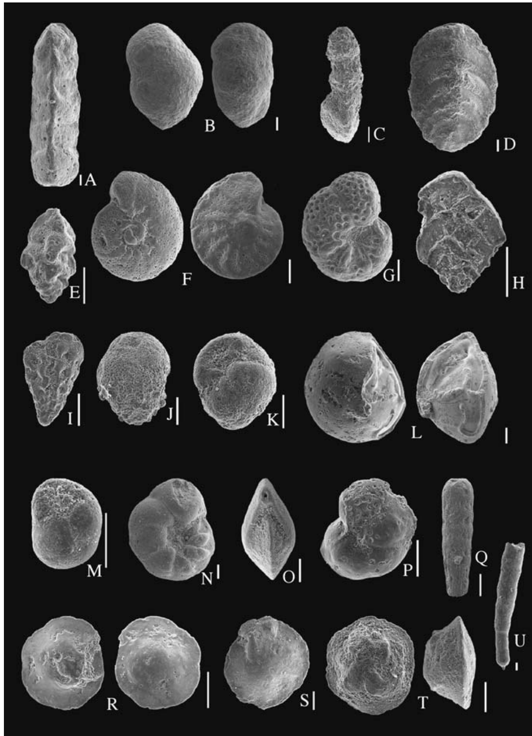
Fig. 10. Scanning electron microscope images of selected small benthic foraminifera from the Agost section. □A. Clavulinoides angularis (metre 82); □B. Gaudryina sp. (metre 84.5); □C. Pseudoclavulina sp. (metre 26.4); □D. Vulvulina sp. (metre 82); □E. Angulogerina muralis (metre 82); □F. Anomalinoidea acutus (metre 90); □G. A. capitatus (metre 5.3); □H. Aragonia aragonensis (metre 84.5); □I. Bolivinoidea crenulata (metre 82.5); □J. Bulimina trinitatensis (metre 102); □K. Buliminella grata (metre 101.7); □L. Cibicoides naranjoensis (metre 84.5); □M. Globocassidulina subglobosa (metre 92); □N. Hanzawaia ammophila (metre 82); □O. Lenticulina sp. (metre 88); □P. Lobatula lobatula (metre 92); □Q. Loxostomoides applini (metre 82); □R. Oridorsalis umbonatus (metre 82); □S. Osangularia plummerae (metre 82); □T. Nuttallides truempyi (metre 101.7); □U. Siphonodosaria annulifera (metre 84.5). Scale bars = 100 \mu m.
