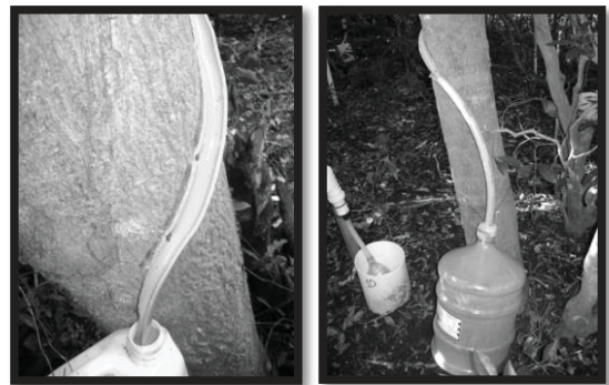
Figura 3 – Coletores utilizados para monitoramento do escoamento pelo tronco
