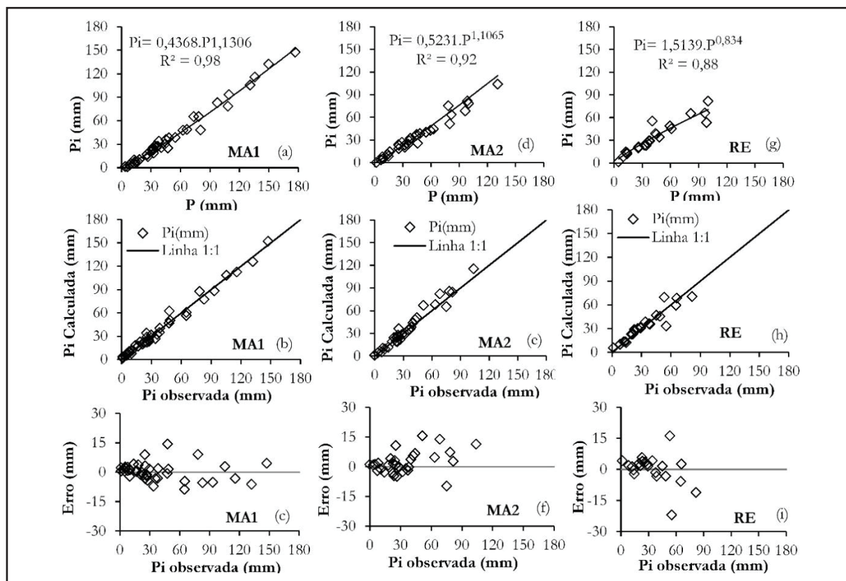
Figura 4 – Ajuste P x Pi nas parcelas MA1 (a), MA2 (d) e RE (g); qualidade do ajuste entre os dados de Pi observados e calculados (linha 1:1) nas parcelas MA1 (b), MA2 (e) e RE (h) e; erro verificado entre os valores de Pi observados e calculados nas parcelas MA1 (c), MA2(f) e RE (i)
