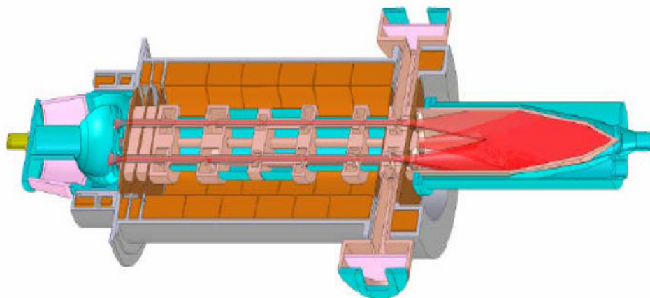
FIGURE 3.4-1. Toshiba E3736 Multi-Beam Klystron.
