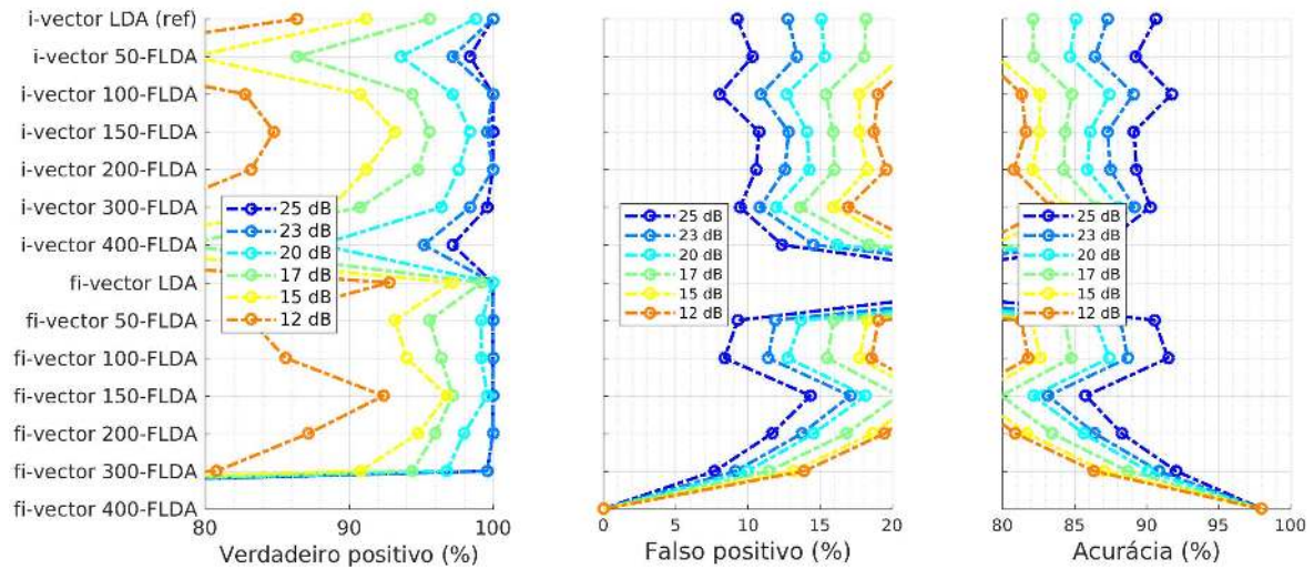
Figura 26 – Taxas de verdadeiro positivo, falso negativo e acurácia para cada metodologia e de acordo com a contaminação SNR do áudio questionado.
