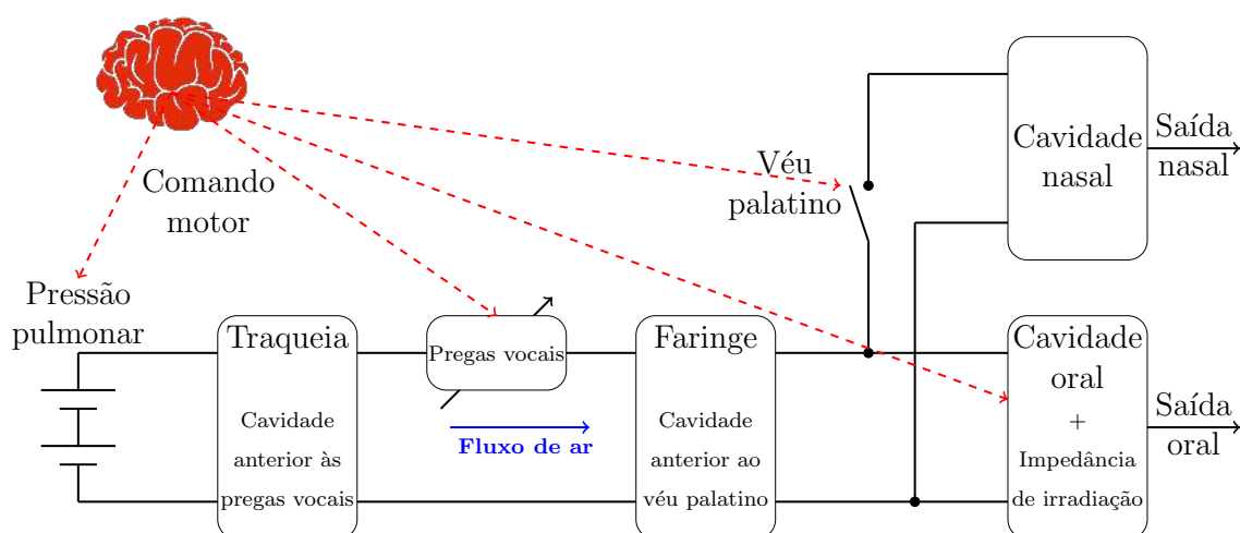
Figura 2 – Diagrama apresentando as etapas do modelo fonte-filtro para produção de vogais. Nesta modelagem a bateria representa a pressão pulmonar sobre os tubos da traqueia, as pregas vocais modulam a pressão subglótica gerando o fluxo de ar que excita os tubos da faringe, trato oral e nasal. Para a produção de outros sons (e.g., fricativas e plosivas), a fonte pode estar em outra região do trato vocal. Adaptado de Fant (1971).
