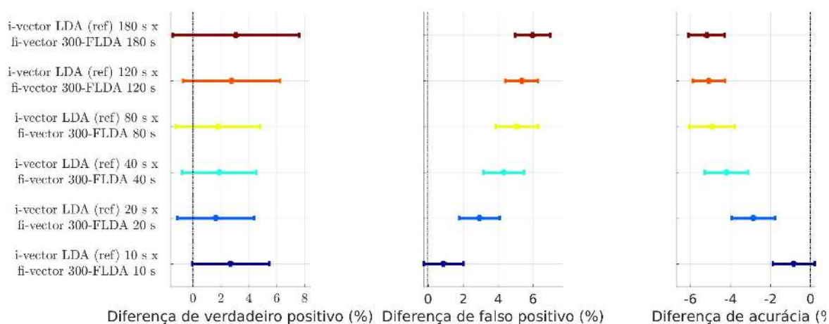
Figura 29 – Análise de variância entre a metodologia de referência e “ fi-vector 300-FLDA ” para as taxas de verdadeiro positivo (à esquerda), falso positivo (centro) e da acurácia (à direita) com \alpha = 0,05 . Em cada linha a diferença média é representada pelo quadrado e o intervalo de confiança, pela linha horizontal.
