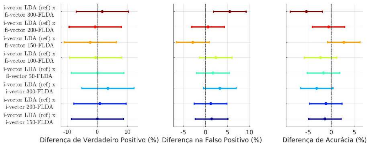
Figura 27 – Análise de variância entre a metodologia de referência e as técnicas que apresentaram melhor desempenho para as taxas de verdadeiro positivo (à esquerda), falso positivo (centro) e da acurácia (à direita) com \alpha = 0,05 . Em cada linha a diferença média é representada pelo quadrado e o intervalo de confiança, pela linha horizontal.
