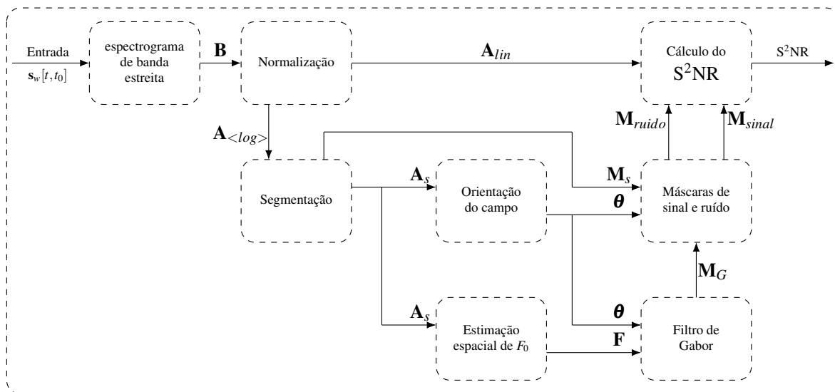
Figura 7 – Etapas do algoritmo S^2NR para obtenção da relação sinal-ruído por quadro s_w[t, t_0] . Fonte: Adaptado de Vieira et al. (2014).
