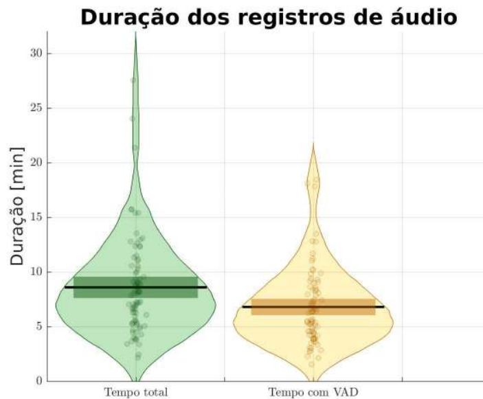
Figura 33 – Gráfico RDI apresentando a duração dos áudios padrão, antes e depois da detecção de atividade de voz. Em cada coluna os pontos são as durações individuais, as curvas laterais são a distribuição de probabilidade empírica, a linha preta horizontal a média e o retângulo escuro é o intervalo de confiança da média para \alpha = 0,05 .
