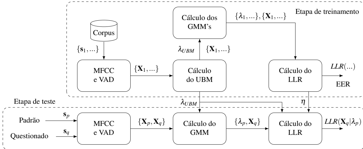
Figura 11 – Etapas da comparação de locutores utilizando GMM-UBM. Primeiramente as características MFCC são extraídas dos registros de voz que são selecionados pelo algoritmo de detecção de atividade de voz (VAD). Destas características são modelados o UBM e as GMM de cada locutor. Na etapa final a pontuação calculada pelo LLR.
