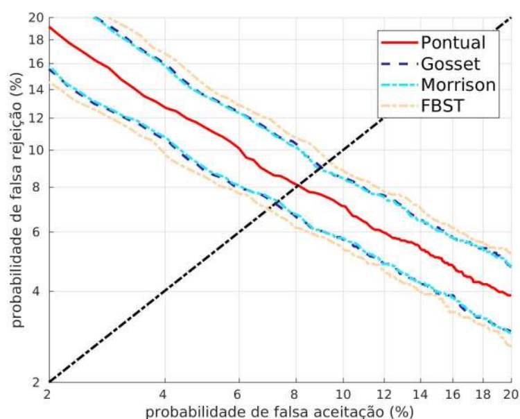
Figura 19 – Curva DET ( detection error tradeoff ) da etapa de treinamento das técnicas de estimativa por intervalo.
