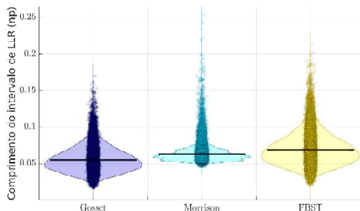
Figura 22 – Gráfico RDI ( Raw data, Description and Inference ) do tamanho de intervalo para cada método de estimativa por intervalo. Nos gráficos, em cada coluna, os pontos são os valores individuais, as curvas laterais indicam a distribuição de probabilidade empírica, a linha preta horizontal a média.
