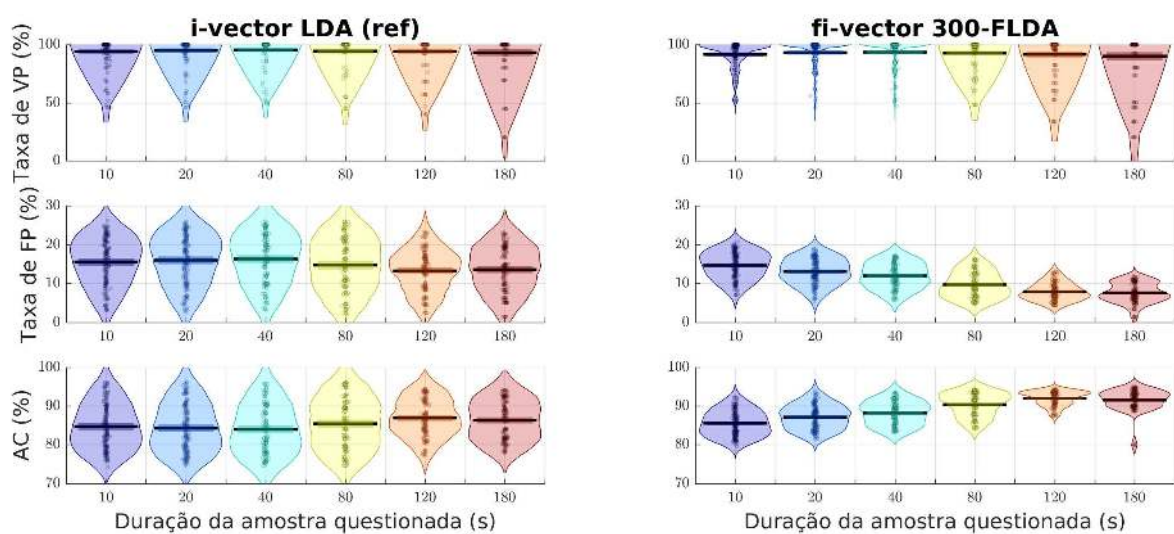
Figura 28 – Curva RDI ( Raw, Description and Inference ) apresentando os valores de verdadeiro positivo (acima), falso positivo (no centro) e acurácia (na base) em relação à duração da amostra questionada. Nos gráficos, em cada coluna, os pontos são os valores individuais, as curvas laterais indicam a distribuição de probabilidade empírica, a linha preta horizontal a média.
