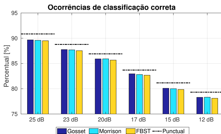
Figura 20 – Percentual de classificações corretas, cenário (a), para cada método de estimativa por intervalo com diferentes valores de SNR na etapa de testes.
