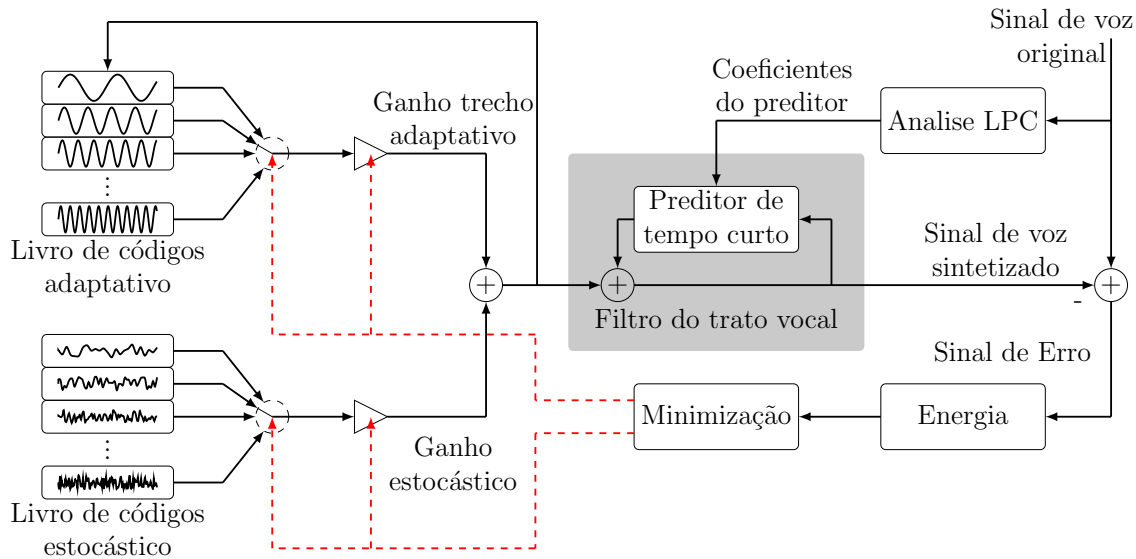
Figura 10 – Predição linear com excitação por código (CELP - Code-excited linear prediction ). Adaptado de (HAUENSTEIN, 2003).
