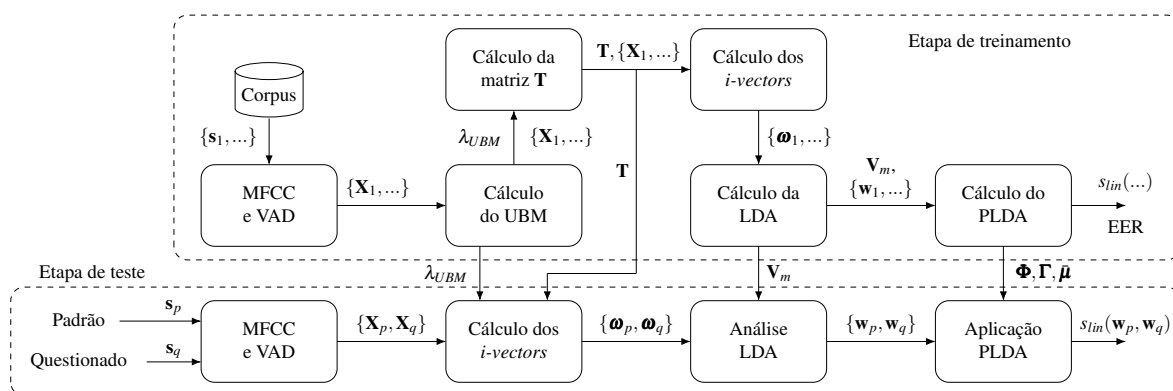
Figura 12 – Etapas da comparação de locutores utilizando i-vector . Primeiramente as características MFCC são extraídas dos registros de voz que são selecionados pelo algoritmo de detecção de atividade de voz (VAD). Destas características são modelados o UBM e a matriz de variabilidade total \mathbf{T} e extraídos os i-vectors . Na etapa final a dimensionalidade é reduzida pela LDA e a pontuação calculada pela PLDA.
