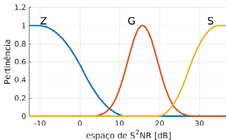
Figura 24 – Conjuntos fuzzy-SNR calculados a partir das amostras padrão da etapa de treinamento. No gráfico a curva “Z” (azul) é localizada entre -10,5 e 12 dB, a “S” (amarela) entre 19,5 e 38 dB, e a Gaussiana (“G” vermelha) centrada em 15,7 com largura (desvio padrão) de 3,7 dB.
