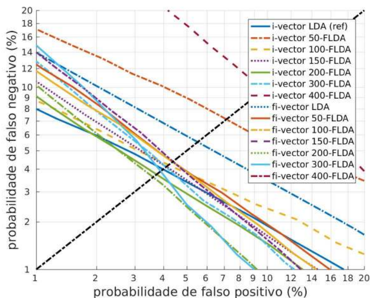
Figura 25 – Curva DET ( Detection Error Tradeoff ) da etapa de treinamento das técnicas de verificação de locutor enumeradas na Tabela 3. Várias técnicas apresentam EER entre 3,5% e 4,5% sendo que apenas três apresentam EER inferior a referência com 4%, sendo elas “ fi-vector 200-FLDA ”, “ i-vector 200-FLDA ” e “ fi-vector 300-FLDA ”.
