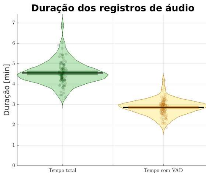
Figura 35 – Gráfico RDI apresentando a duração dos áudios do Corpus CEFALA-1 antes e depois do processamento VAD. Em cada coluna os pontos são as durações individuais, as curvas laterais são a distribuição de probabilidade empírica, a linha preta horizontal a média e o retângulo escuro é o intervalo de confiança da média para \alpha = 0,05 .
