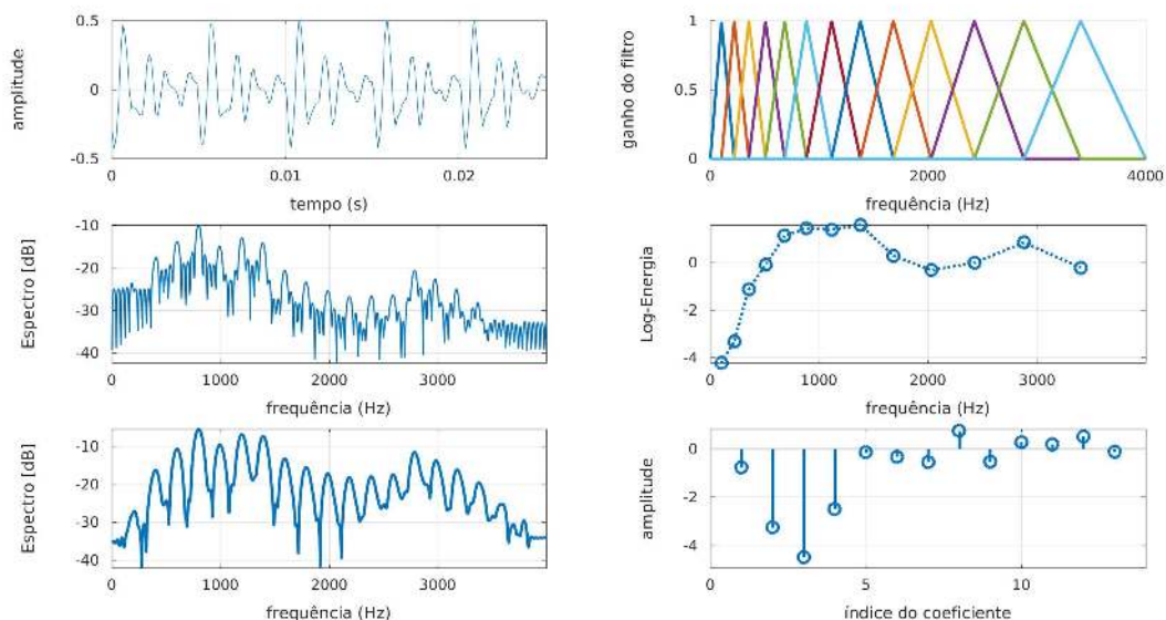
Figura 6 – Exemplo indicando as etapas do processamento para obtenção dos MFCC. No painel superior esquerdo tem-se o sinal de áudio, no painel logo abaixo tem-se o espectro de magnitude sem o janelamento e a pré-ênfase, no painel inferior esquerdo o espectro de magnitude utilizando a janela de Hamming e pré-ênfase. No painel superior direito têm-se os filtros triangulares, logo abaixo o logaritmo da energia para cada banda crítica, e, no painel inferior direito, os MFCC. Adaptado de (HANSEN; HASAN, 2015).
