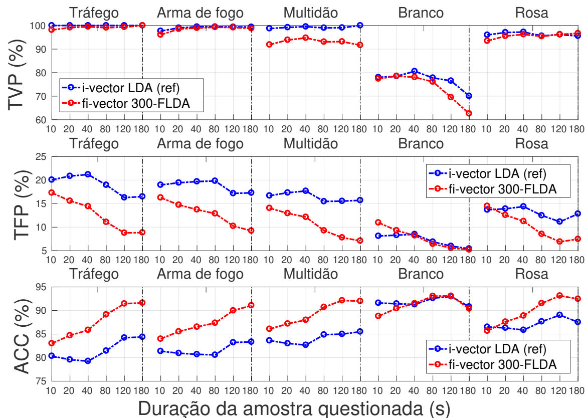
Figura 30 – Média das taxas de verdadeiro positivo (TVP) no painel acima, falso positivo (TFP) ao centro e acurácia (ACC) abaixo em relação à duração da amostra questionada pelo tipo de ruído. Da esquerda para direita são agrupados os resultados de acordo com o tamanho da amostra questionada (eixo horizontal inferior) para cada tipo de ruído contaminante (eixo horizontal superior).
