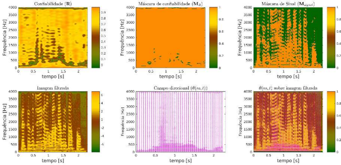
Figura 9 – Exemplo indicando as etapas finais do processamento para obtenção do S^2NR . No painel superior direito tem-se a matriz de confiabilidade \mathbf{R} e, à sua direita, a máscara de confiabilidade \mathbf{M}_R(m,t) . No painel superior direito tem-se a máscara de sinal \mathbf{M}_{sinal} . Na porção inferior tem-se a imagem filtrada seguida da orientação ângulo \theta(m,t) e, no painel inferior direito, a orientação de ângulo sobre o espectrograma.
