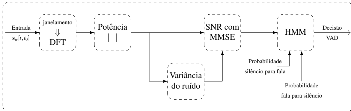
Figura 4 – Etapas do algoritmo para detecção de atividade de voz proposto por Sohn et al. (1999). O sinal \mathbf{s}[t] é dividido em quadros para o cálculo da DFT, do espectro de potência estima-se a variância do ruído e a SNR minimizando o erro quadrático médio (MMSE). Estes parâmetros, juntamente com as probabilidades de transição entre fala para silêncio (e vice-versa), alimentam um HMM para tomada de decisão. Adaptado de (KIZHANATHAM, 2003, p. 10)
