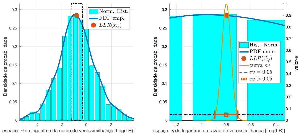
Figura 17 – Exemplo da estimativa por intervalo sobre a média de LLR(x_Q) . O painel à esquerda mostra o histograma normalizado de LLR(x_Q) ocorrências e a função de densidade de probabilidade empírica (linha grossa). No mesmo painel, o retângulo tracejado indica a região mostrada no painel à direita. Neste painel, a linha sólida amarelo escuro em forma de sino indica curva ev e a barra de erro laranja na horizontal indicam intervalo de evidência e a média amostral.
