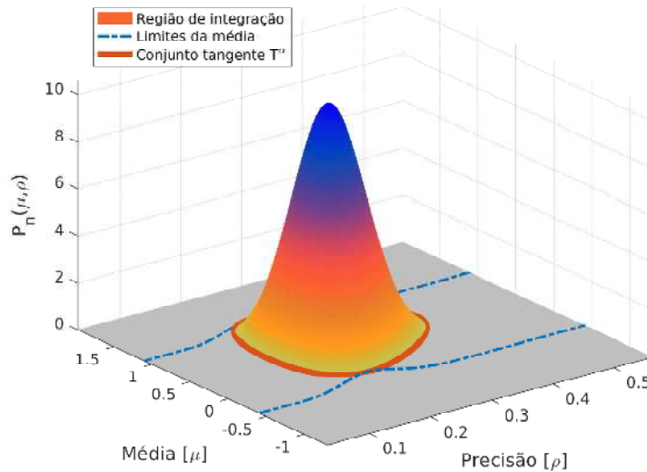
Figura 15 – Exemplo de conjunto T^{0,05} , ou seja \alpha = 0,05 , que delimita a superfície de integração. Na imagem, a linha vermelha, paralela ao plano horizontal, indica o conjunto T^{0,05} , a porção da curva em degradê está contida no conjunto e as linhas azuis são os limites superior e inferior do conjunto no eixo da média \mu .
