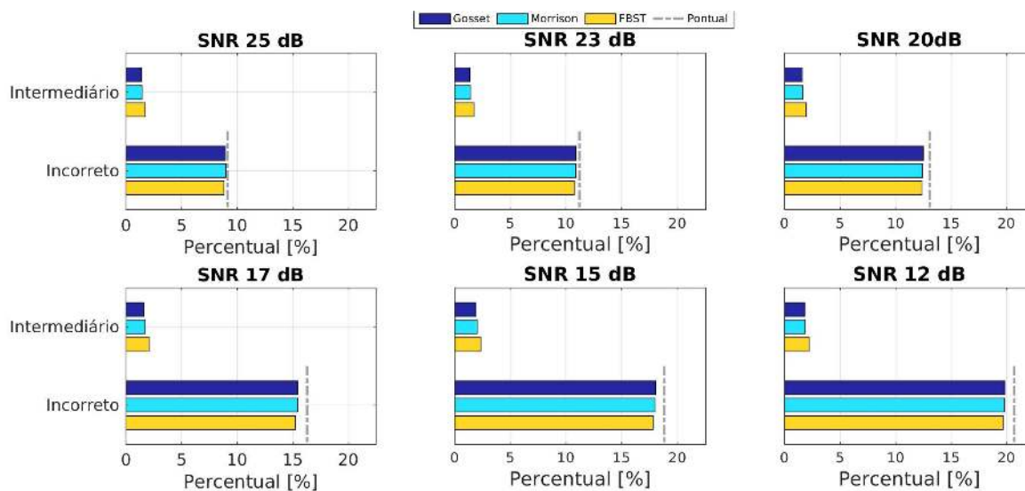
Figura 21 – Resultados da estimativa por intervalo apresentando o percentual de ocorrências dos cenários (b) e (c) da Figura 18. As barras horizontais indicam as porcentagens por método, enquanto a linha vertical tracejada em cinza escuro indica a porcentagem de erro da inferência pontual.
