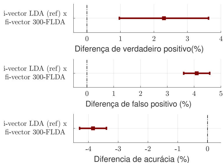
Figura 32 – Análise de variância entre o método de referência e “ fi-vector 300-FLDA” as taxas de verdadeiro positivo (acima), falso positivo (centro) e da acurácia (abaixo), com \alpha = 0,05 , considerando apenas os resultados com a duração da amostra questionada. Em cada linha a diferença média é representada pelo quadrado e o intervalo de confiança, pela linha horizontal.
