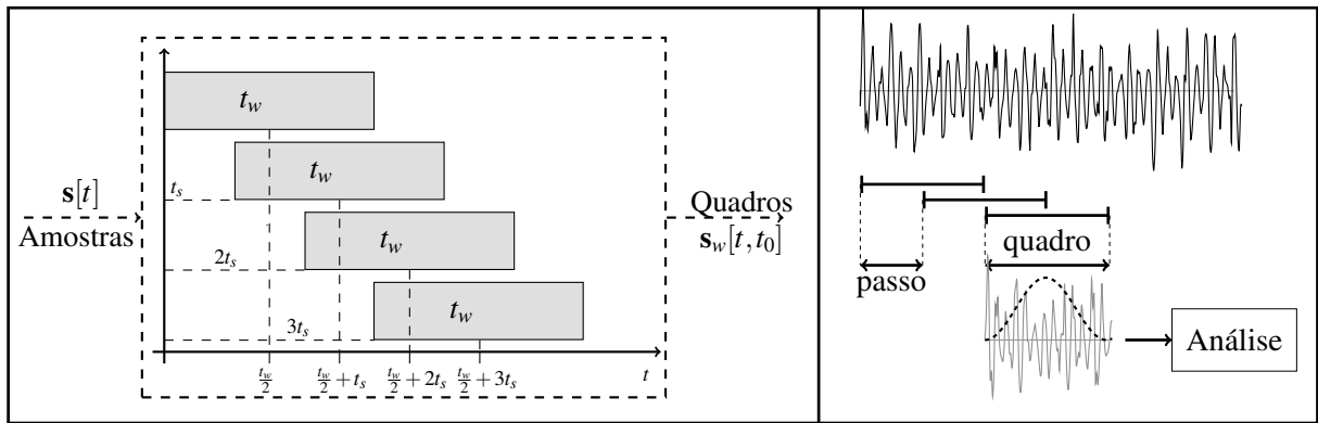
Figura 3 – Diagramação do processo de separação dos quadros de voz, indicando o comprimento da janela t_w , e o passo de tempo t_s .
