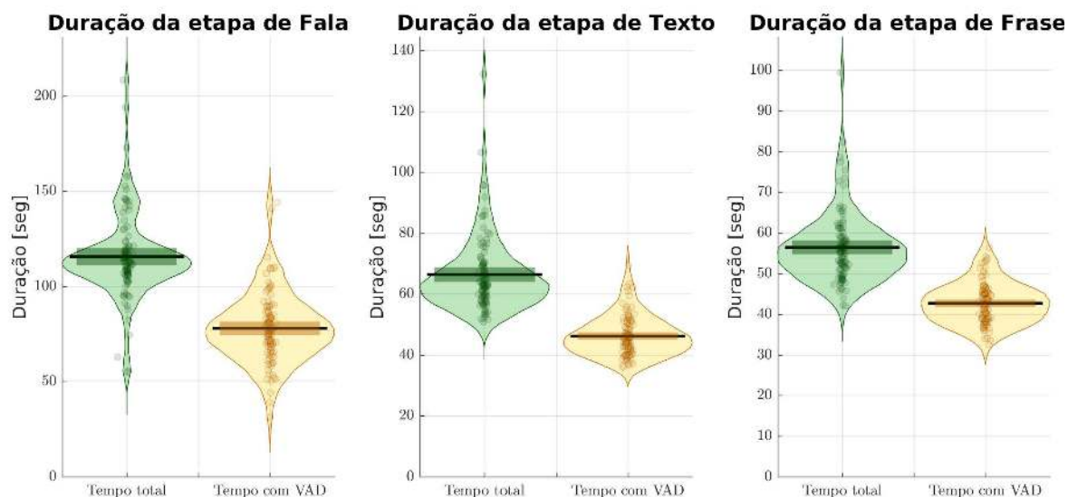
Figura 36 – Gráfico RDI apresentando a duração das etapas dos áudios do Corpus CEFALA-1 antes e depois do processamento VAD. Em cada coluna os pontos são as durações individuais, as curvas laterais são a distribuição de probabilidade empírica, a linha preta horizontal a média e o retângulo escuro é o intervalo de confiança da média para \alpha = 0,05 .
