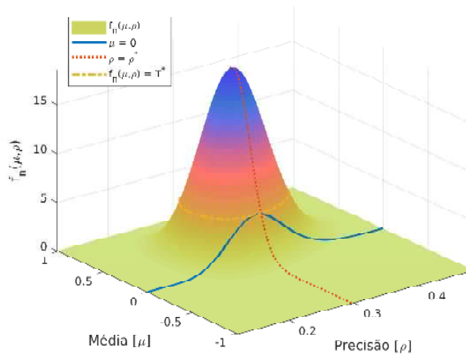
Figura 13 – Função densidade de Probabilidade f_n(\mu, \rho | n, \bar{x}, Q) . Na imagem a linha azul f_n(\mu = 0, \rho) indica a hipótese nula. O valor máximo sobre a linha azul é f_n^* = f_n(\mu = 0, \rho_A) que define o contorno da linha amarela onde f_n(\mu, \rho) = f_n^* que delimita o conjunto tangente T^* onde f_n(\mu, \rho) \geq f_n^* . A linha vermelha indica o subconjunto f_n(\mu, \rho = \rho^*) que atravessa o valor \rho^* . Adaptado de Arruda (2012).
