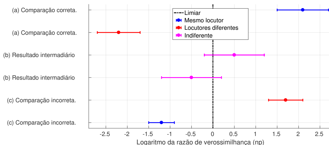
Figura 18 – Cenários de resultados da estimativa por intervalo. A linha pontilhada vertical indica o limiar de decisão em LLR = 0 , pontuação acima do limiar associa locutores e abaixo desassocia. As linhas azuis representam as comparações entre áudios de um mesmo falante e as vermelhas entre falantes diferentes. Os cenários são o de comparação correta (a), de resultados intermediários (b), e de comparações incorretas (c).
