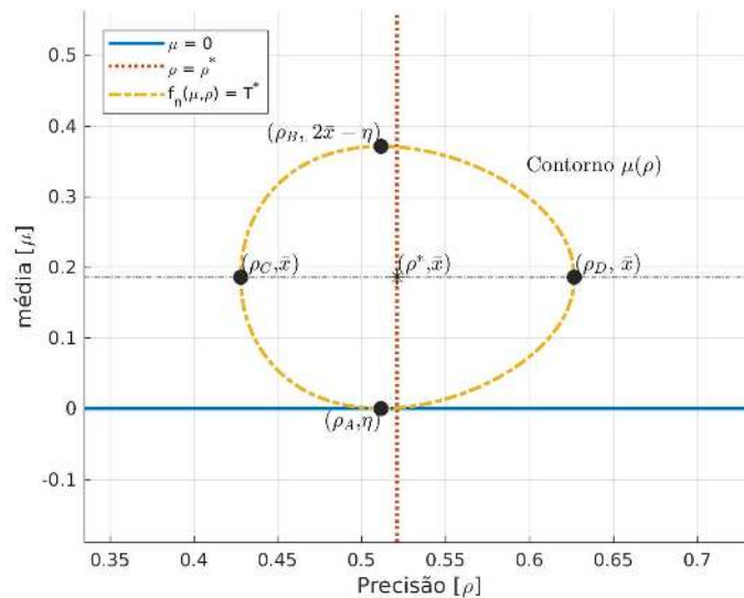
Figura 14 – Contorno e pontos extremos do conjunto tangente T^* .
