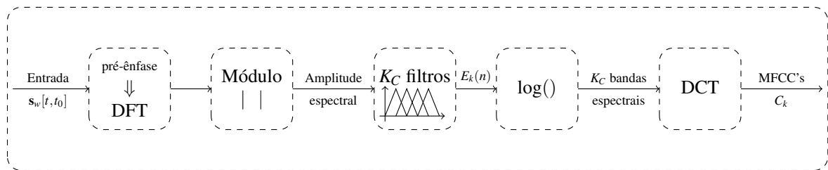
Figura 5 – Etapas na obtenção dos componentes mel-cepstrais com filtro triangular.
