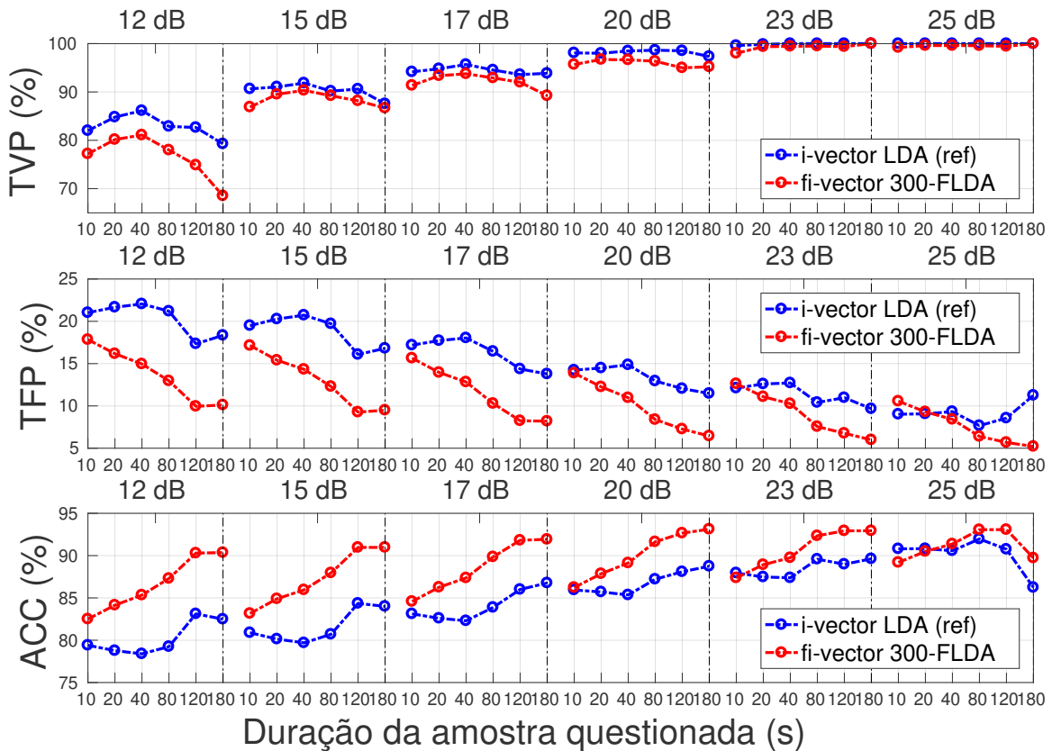
Figura 31 – Médias das taxas de verdadeiro positivo (acima), falso positivo (no centro) e acurácia (na base) em relação à duração da amostra questionada e a intensidade do ruído para o método de referência e para “ fi-vector 300-FLDA ”. Da esquerda para direita são agrupados os resultados de acordo com o tamanho da amostra questionada (eixo horizontal inferior) para a intensidade do ruído contaminante (eixo horizontal superior).
