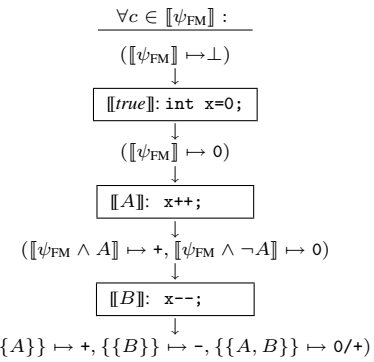
(d) Using the shared simultaneous analysis, \mathcal{A}4 .
