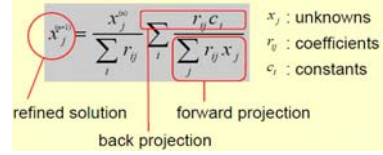
Fig. 1. Interpretation of the update law in EM
