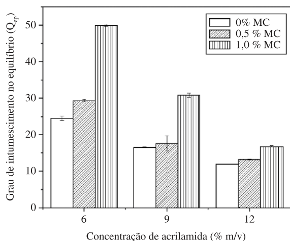
Figura 2. Dependência dos valores de grau de intumescimento no equilíbrio ( Q_{eq} ) em função da concentração de acrilamida para os hidrogéis de PAAm-MC com diferentes composições a 25,0 \pm 0,1 °C.
