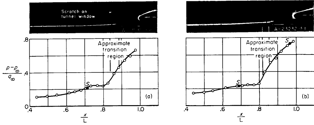
(a) S-9; M_\infty=0.47 ; \alpha=-4^\circ ; R_L=0.47 \times 10^6 . (b) S-9; M_\infty=0.76 ; \alpha=-4^\circ ; R_L=0.50 \times 10^6 .
