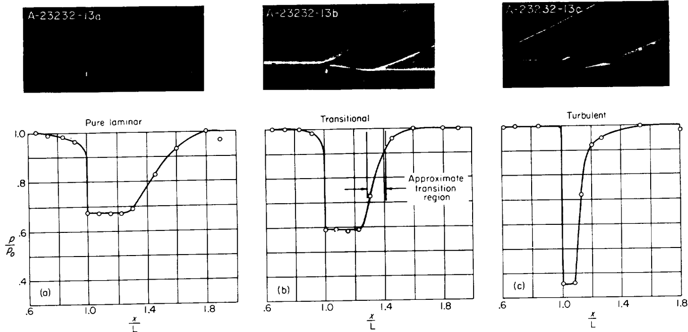
(a) B-2; M_o=2.0 ; R_L=0.17 \times 10^6 . (b) B-2; M_o=2.0 ; R_L=0.50 \times 10^6 . (c) B-1-c (trip 1); M_o=2.0 ; R_L=0.39 \times 10^6 .
