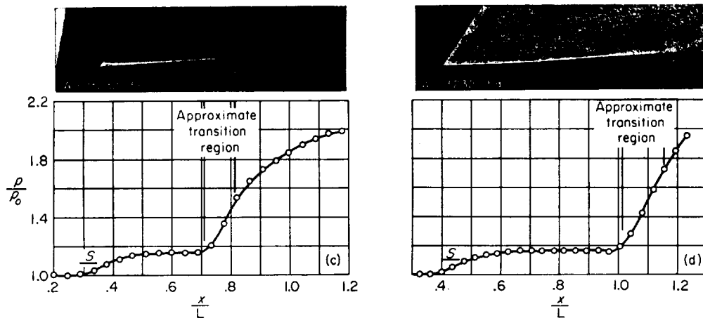
(c) CC10°-2; M_0=1.4 ; R_L=0.33 \times 10^6 . (d) CS25°-1; M_0=1.7 ; R_L=0.26 \times 10^6 .
