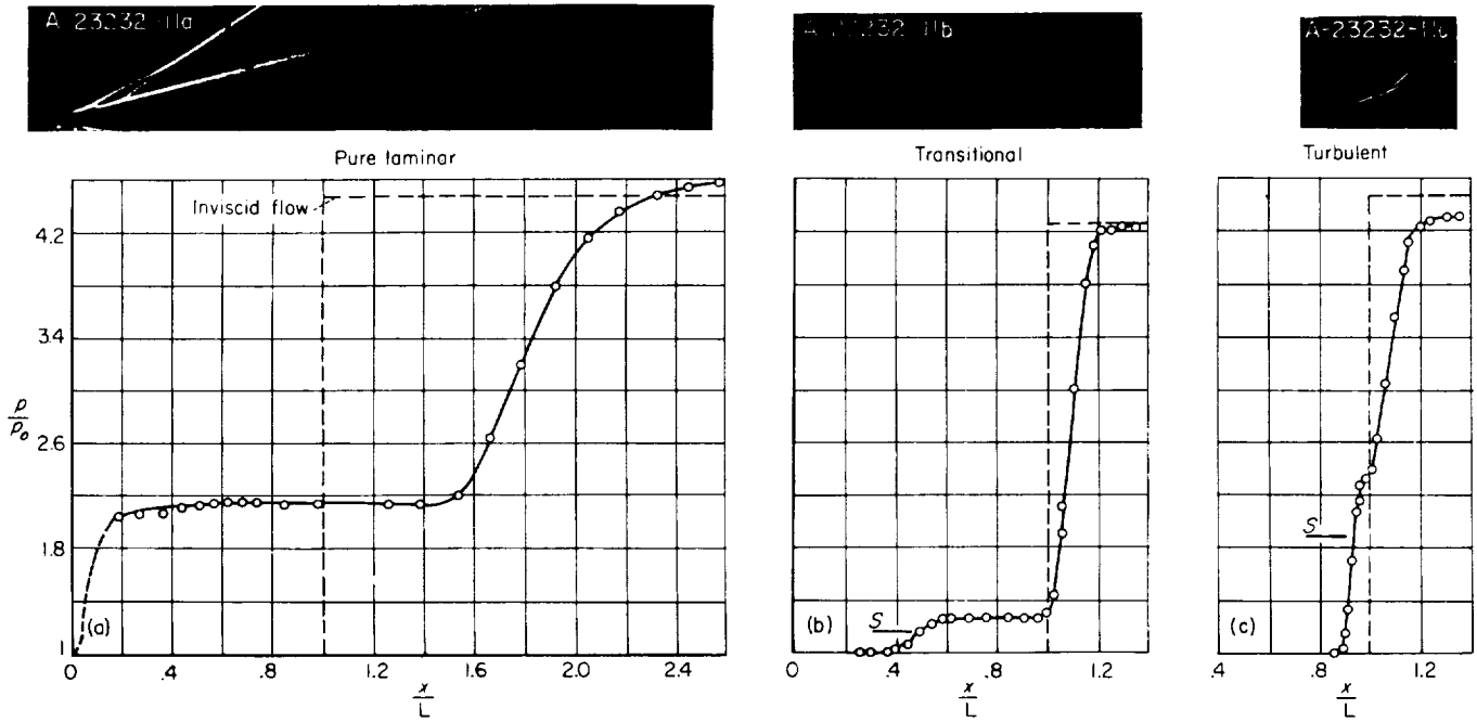
(a) CC25°-2; M_\infty=2.7 ; R_L=0.033 \times 10^6 . (b) CC25°-4; M_\infty=2.6 ; R_L=0.33 \times 10^6 . (c) CC25°-5 (trip 4); M_\infty=2.7 ; R_L=1.65 \times 10^6 .
