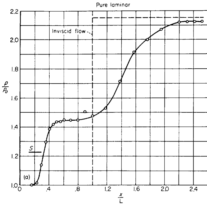
(a) 16.5^\circ-1 ; M_o=2.4 ; R_L=0.054 \times 10^6 .
