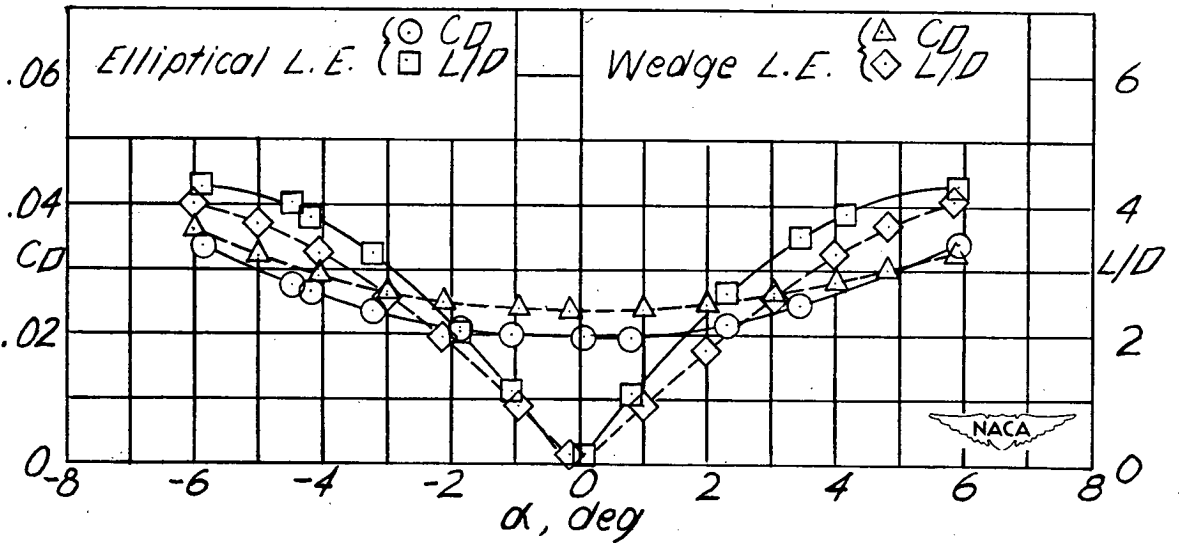
(d) Wing 4. w=1.017 ; R=860,000 .
