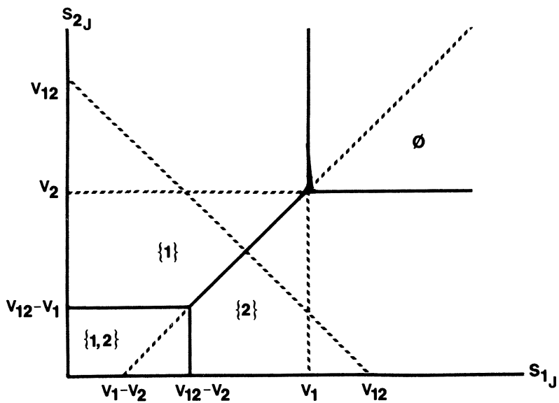
FIGURE 1—Subadditive case.
