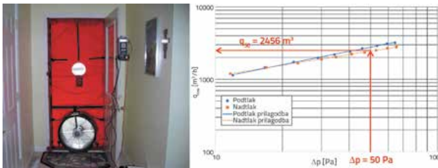
Slika 21. Blower door uređaj te prikaz rezultata mjerenja
