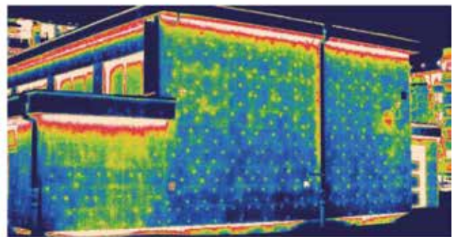
Slika 11. Shematski prikaz povećanog toplinskog toka zbog promjene materijala i geometrije građevnog dijela (lijevo) [12], termogram vanjske ovojnice zgrade s izraženim linijskim i točkastim toplinskim mostovima (desno) [13]
