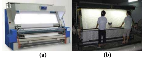
Şekil 2. Offline kumaş hatası tespit sistemleri (a) Makine odaklı kumaş kontrolü (b) İnsan odaklı kumaş kontrolü [7] (Offline fabric error detection systems: (a) machine-based fabric control, (b) manual fabric control)
