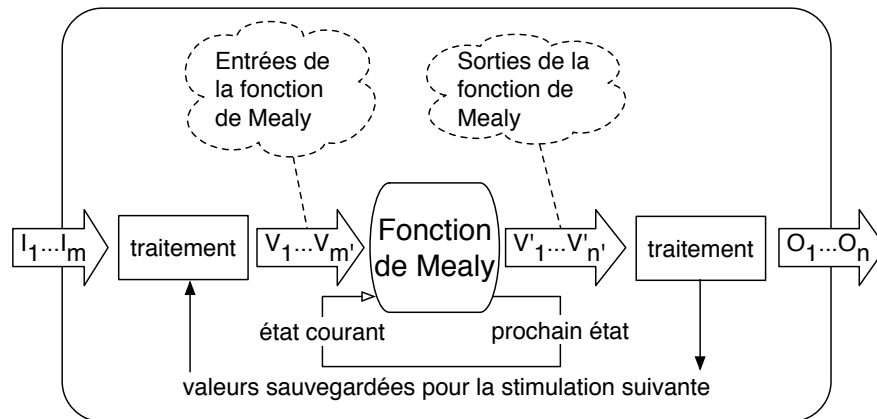
Figure 4.1: Processus asynchrone coquille général
