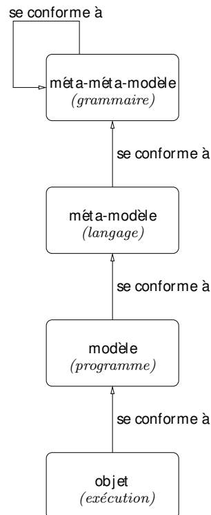
Figure 1.1: Hiérarchie des modèles dans l'approche IDM
