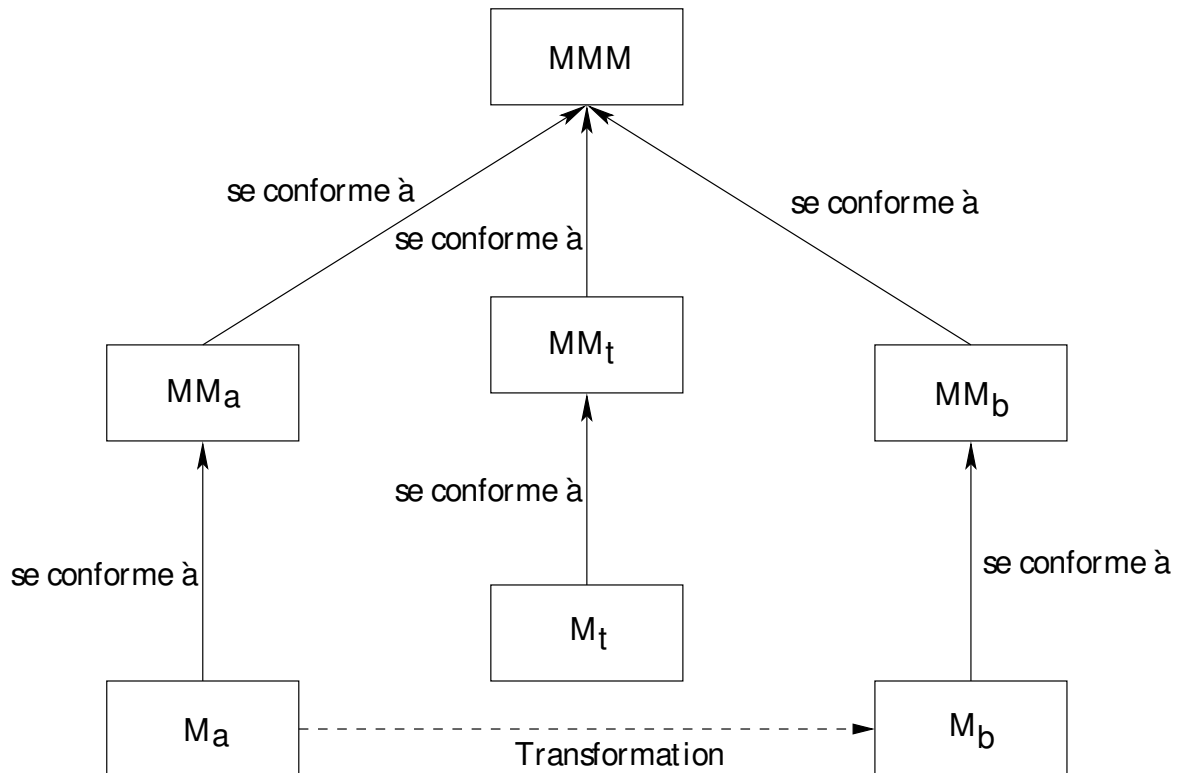
Figure 1.8: Schéma des transformations de modèles dans l'approche QVT
