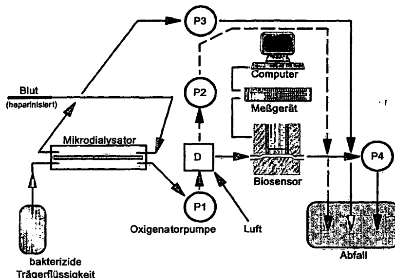
Abb. 4 Fouling-resistentes Meßsystem mit Oxigenatorpumpe zur Carrier-Analyse von \beta -D-Glucose oder L-Lactat im heparinisierten Blut mit O_2 -sensitiv-enzymatischen Membranelektroden.
