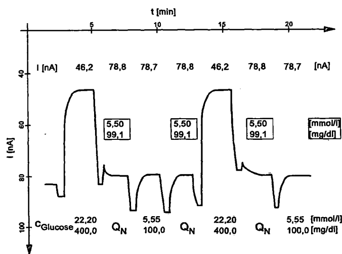
Abb. 2 Durchflußmessung von \beta - D -Glucose im 1 : 21 verdünnten Richtigkeits-Kontrollserum Qualitrol N ® (Q N ) mit einem O_2 -sensitiv-enzymatischen Biosensor (Membran SBC-1010). Umrahmt ist die jeweils aus Zweipunktkalibrierung errechnete Glucosekonzentration in Q N . Die den Glucosekonzentrationen zuzuordnenden Stromstärken sind jeweils oberhalb der Meßkurve aufgeführt. Glucose in Qualitrol N ® der Chargen-Nr. 390 laut Datenschlüssel (E. Merck, Darmstadt):
