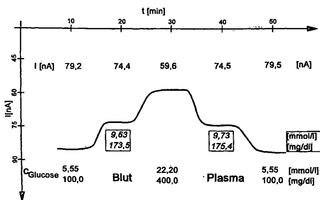
Abb. 5 Ausschnitt aus 6,5 Stunden kontinuierlicher Hämooanalytik der \beta -D-Glucose nach dem Prinzip der Zwischenträgeranalyse mit Oxigenatorpumpe und O_2 -sensitiv-enzymatischer Membrandurchflußelektrode (Membran SBC-1010). Umrahmt ist die jeweils aus Zweipunktkalibrierung errechnete Glucosekonzentration in Blut und dessen Plasma. Beachte die vernachlässigbaren Konzentrationsunterschiede bei dieser Analysen-Methode, hierüber werden wir separat berichten. Die den Glucosekonzentrationen zuzuordnenden Stromstärken sind jeweils oberhalb der Meßkurve aufgeführt.
