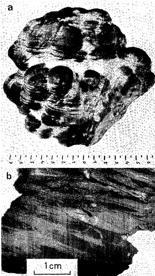
Fig.3. Poupée d'oxydes de fer et de manganèse accolée aux bancs minéralisés. Schiste imprégné d'oxydes
