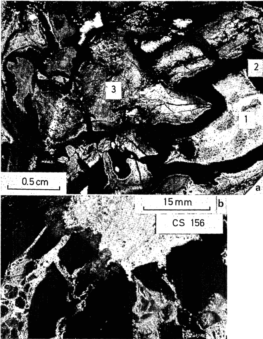
Fig.9. a) Minéral associé à la cuirasse bauxitique. 1: Poche de kaolinite et gibbsite. 2: Cortex concrétionné de lithiophorite secondaire. 3: Schiste imprégné d'oxydes de fer et de manganèse. b) Minéral bréchique à ciment gibbsitique (dont des veinules de gibbsite bien cristallisée)
