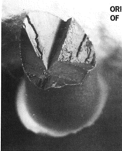
760°C (1400°F)
