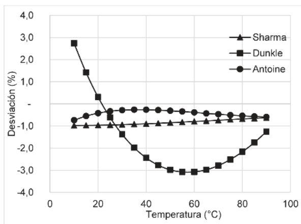
Figura 4. Desviación porcentual de la presión de vapor del agua calculada según las correlaciones de Dunkle, Antoine y Sharma-Mullick (Keenan-Keyes).
