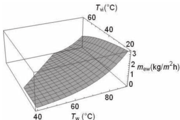
Figura 11. Productividad de destilado calculada empleando los números adimensionales, en función de las temperaturas del agua T_w y del vidrio T_v .
