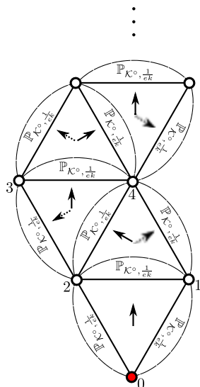
FIG 17. The Benjamini–Schramm limit of random k -trees.
