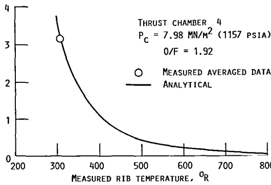
(D) SOOT THICKNESS 31.8 (12.5 IN.) FROM INJECTOR FACE.
