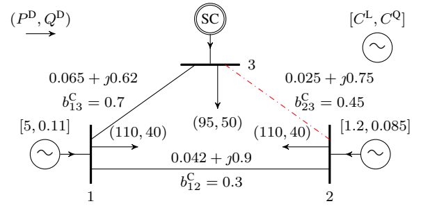
Fig. 5. LMBM3 3-bus system.
