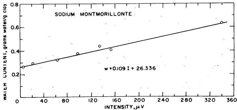
b. Sodium-montmorillonite.
