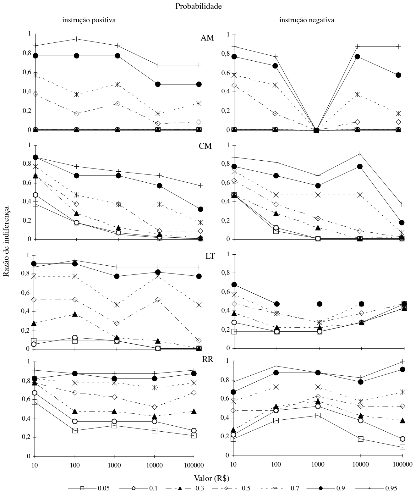
Figura 1. Razão de indiferença como função da magnitude da quantia provável com instrução positiva e negativa para os participantes AM, CM, LT e RR. Curvas diferentes apresentam os resultados de cada probabilidade utilizada.
