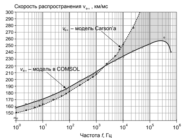
Рис. 10. Зависимость величины скорости распространения электромагнитной волны в канале «фаза-земля» для различных частотных компонент фронта ЭМВ
