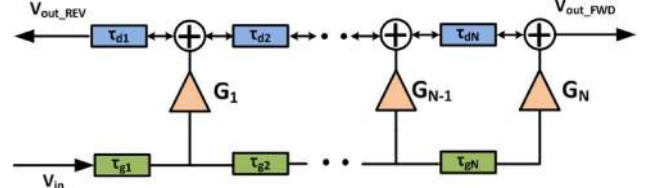
Fig. 14. N -stage DA.
