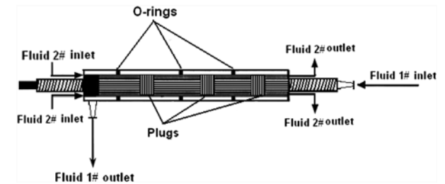
Fig. 3. Fabric woven module.
