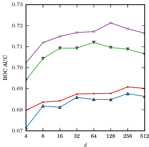
(b) MovieLens
