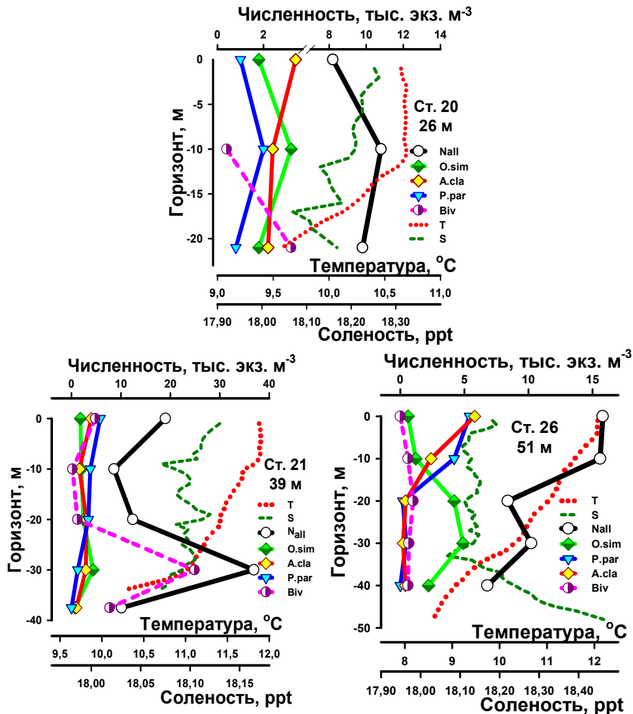
Рис. 4. Вертикальное распределение температуры воды (Т), солёности (S) и численности разных групп и видов ММЗП в водах юго-восточного побережья Крыма: Феодосийского залива (ст. 20 и 21) и Карадага (ст. 26). Обозначения см. рис. 2
