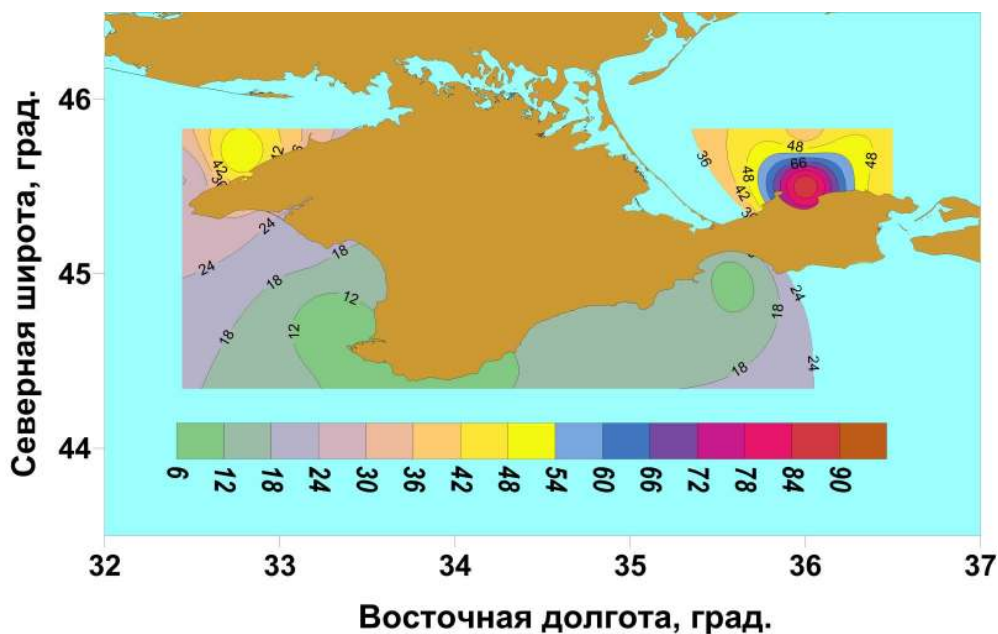
Рис. 1. Расположение станций 84-й экспедиции НИС «Профессор Водяницкий» и пространственное распределение общей численности метазойного микрозоопланктона (тыс. экз. м -3 ) в поверхностном слое (вверху) и на глубине ~10 м (внизу) в черноморских и азовоморских водах Крыма в апреле 2016 г. Во врезке – расположение станций в водах южного берега Крыма в районе бухты Ласпи
