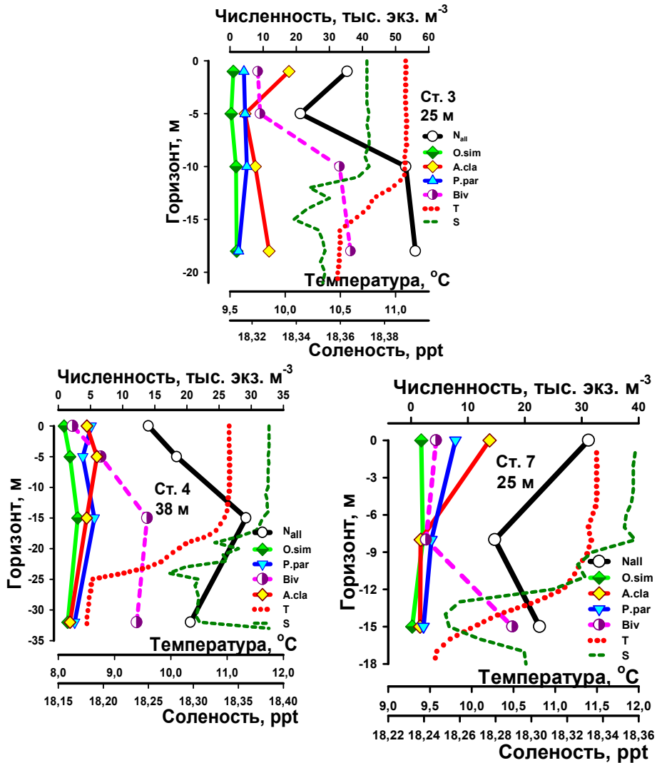
Рис. 2. Вертикальное распределение температуры воды (Т), солености (S) и численности разных групп и видов ММЗП в водах западного побережья Крыма: Каркинитского (ст. 3 и 4) и Каламитского (ст. 7) заливов. N_{all} – общая численность ММЗП; O.sim – численность Oithona similis ; A.cla – численность Acartia clausi ; P.par – численность Paracalanus parvus ; Biv – численность велигеров Bivalvia
