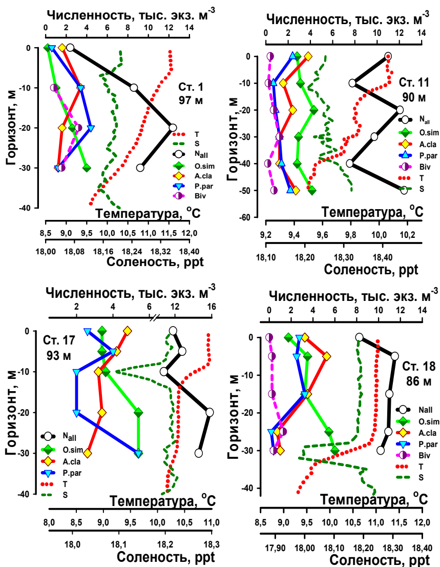
Рис. 3. Вертикальное распределение температуры воды (Т), солёности (S) и численности разных групп и видов ММЗП в водах севастопольского побережья (ст. 1) и южного берега Крыма (ст. 11, 17 и 18). Обозначения см. рис. 2
