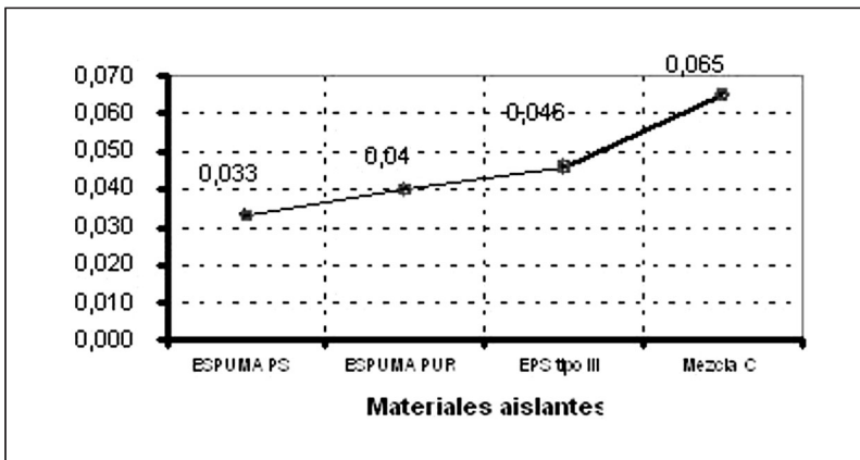
Gráfica 6. Conductividad térmica de algunos materiales aislantes comparados con la conductividad de la mezcla C.
