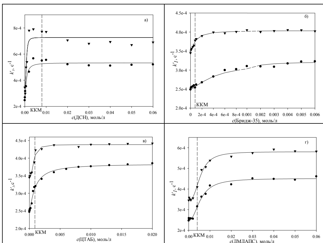
Рисунок 1. Зависимость константы скорости псевдопервого порядка взаимодействия МЗ (●) и БЗ (▼) с водой от концентрации ПАВ: а) ДСН, б) Бридж-35, в) ЦТАБ, г) ДМДАПС, t = 25 °С, \text{pH} = 3 , раствор содержит 1.0 % об. ацетонитрила. На рисунке б) абсцисса имеет различный масштаб до 0.001 моль/л и после этого значения. Линии проведены в соответствии с уравнением модели Пишкевича. Пунктиром обозначена область ККМ соответствующего ПАВ.
