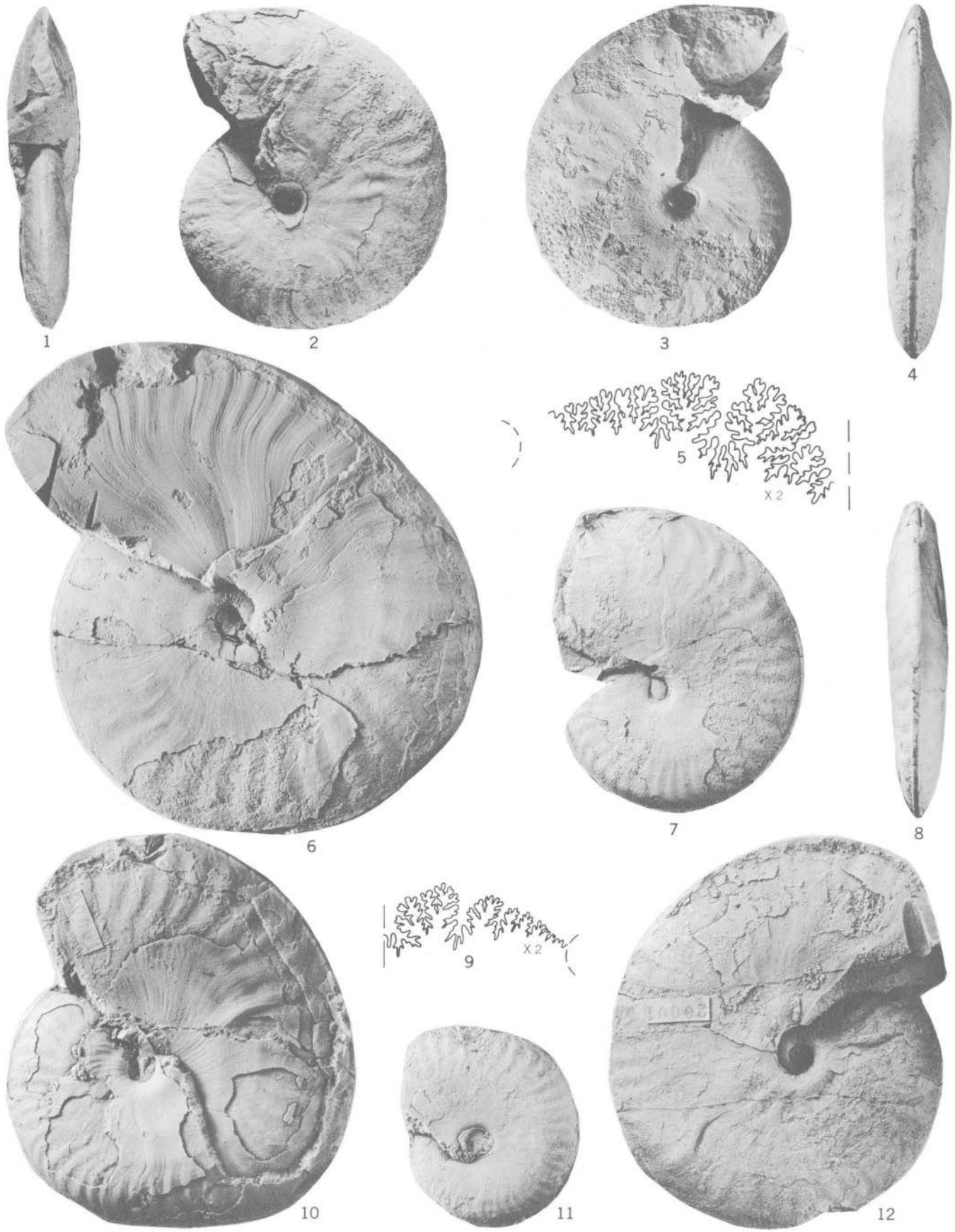
OPPELIA (LIROXYITES)
