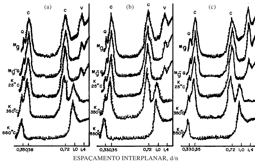
Figura 2. Difratoigramas da fração argila do perfil 2 (PVAe). (a) horizonte AB; (b) horizonte 2Bt2 e (c) horizonte 2BC. Q: quartzo; C: caulinita; V: vermiculita. Valores de d/n em nanômetros.
