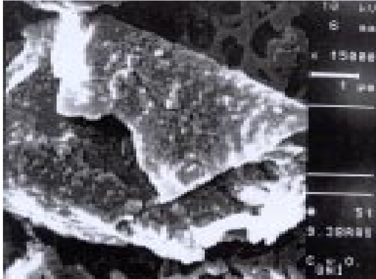
Figura 6. Fotografia obtida por microscopia eletrônica de varredura, mostrando pseudomorfozes de montmorilonita, para caulinita, no horizonte 2Btn do perfil 9 (SXen).
