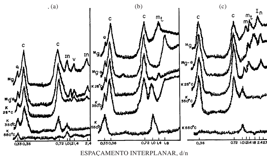
Figura 3. Difratoigramas da fração argila do perfil 9 (SXen). (a) horizonte Ap; (b) horizonte 2Btn e (c) horizonte 2Cr2. Q: quartzo; C: caulinita; V: vermiculita; In: interestratificado; Mt: montmorilonita. Valores de d/n em nanômetros.
