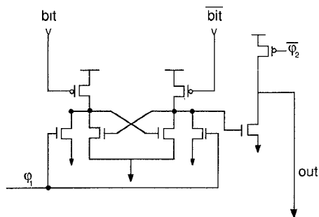
Fig. 8. RAM sense amplifier.
