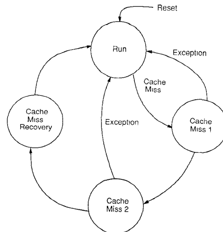
Fig. 14. Cache-miss FSM.
