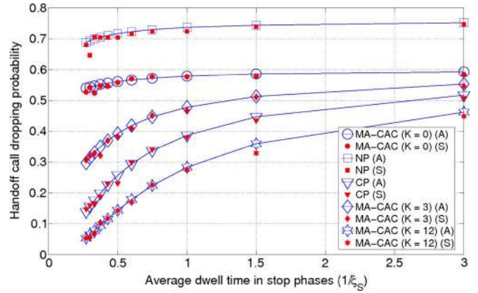
Fig. 14. HCDP versus 1/\xi_S ( \lambda_N = 16 ).
