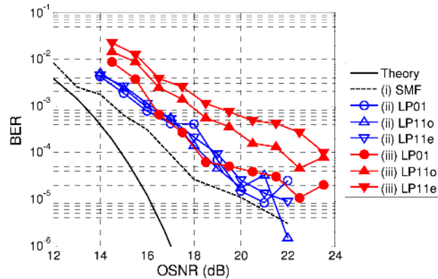
Fig. 8. BER vs. OSNR.
