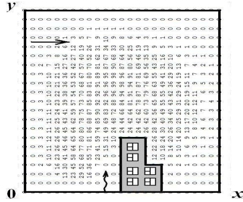
Рис. 7. Зона загрози зараження для моменту часу t = 5,49 с (повітряна завіса на відстані 4,5 м від будинку, швидкість повітряної струї 10 м/с)
