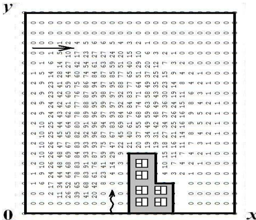
Рис. 6. Зона загрози зараження для моменту часу t = 4,09 с (повітряна завіса на відстані 4,5 м від будинку, швидкість повітряної струї 10 м/с)
