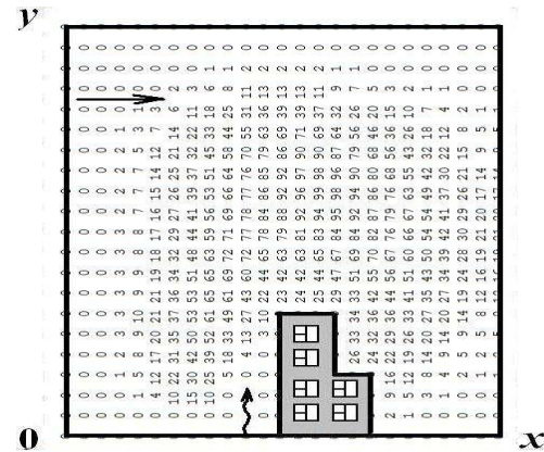
Рис. 8. Зона загрози зараження для моменту часу t = 7,39 с (повітряна завіса на відстані 4,5 м від будинку, швидкість повітряної струї 10 м/с)
