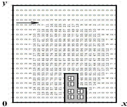
Рис. 5. Розподіл концентрації небезпечного речовини при відсутності повітряної завіси, t = 7,39 с
