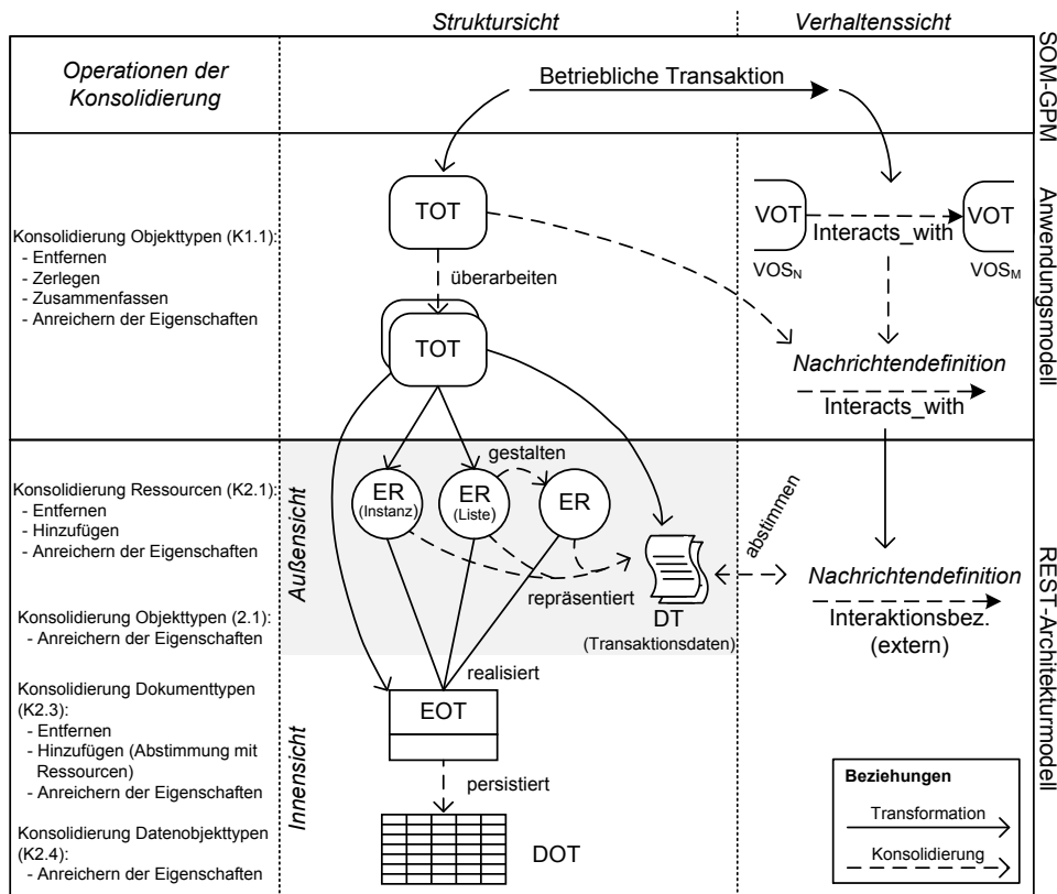
Abbildung 5.23: Beziehungen zwischen der betrieblichen Transaktion und der RESTful SOA
