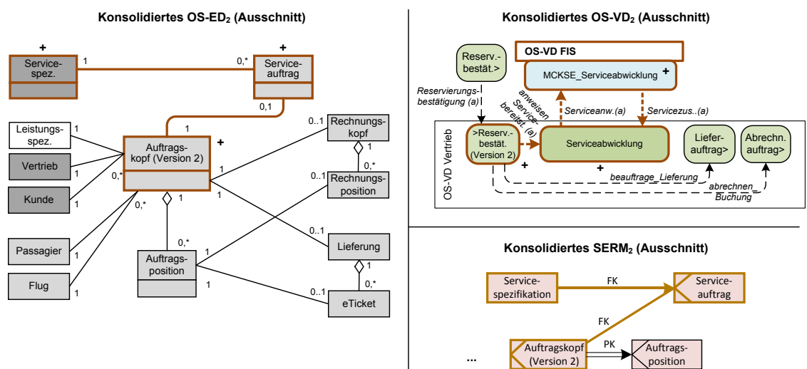
Abbildung 6.28: Konsolidiertes OS-ED 2 und Ausschnitt des konsolidierten OS-VD 2 (Szenario FIS)
