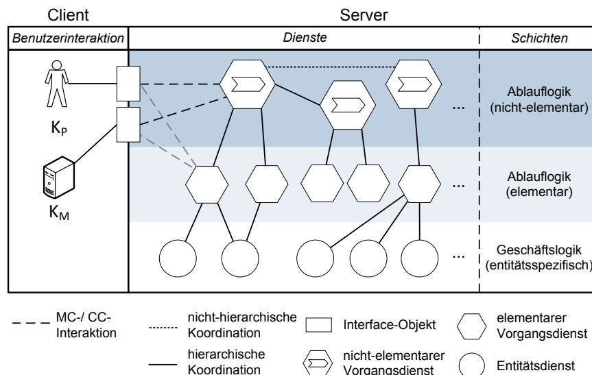
Abbildung 3.6: Schichtenmodell der RESTful SOA
