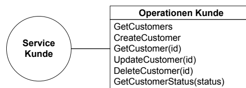
Abbildung 3.4: Anwendungsspezifische Schnittstelle des Service Kunde (in Anlehnung an [Tilk07, S. 399])
