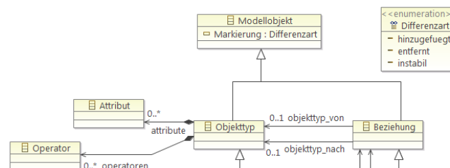
Abbildung 7.8: Metamodell des Überarbeitungsschemas der fachlichen AwS-Spezifikation (Ausschnitt)
