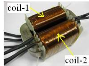
(d) Coupled inductor in 2 nd stage
