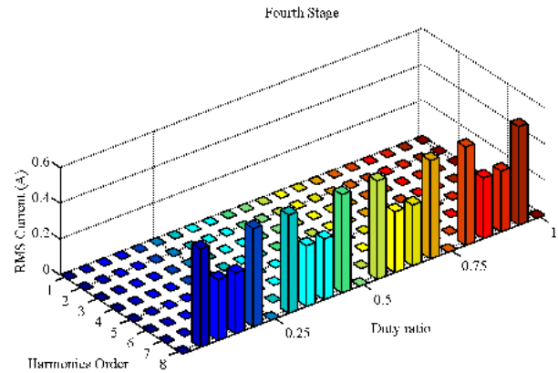
(d) Harmonics components in the stage-4 current
