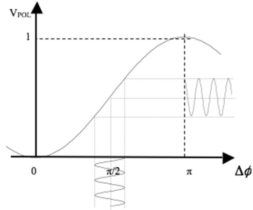
Figura 2. Curva de transferencia de potencia de un modulador MZ. Fuente: Los autores
