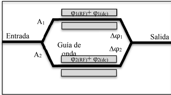
Figura 1. Modulador MZ con control doble. Fuente: Los autores
