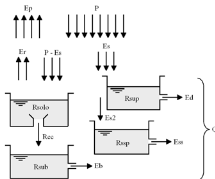
Figura 1 - Ilustração do modelo diário SMAP de quatro reservatórios.
